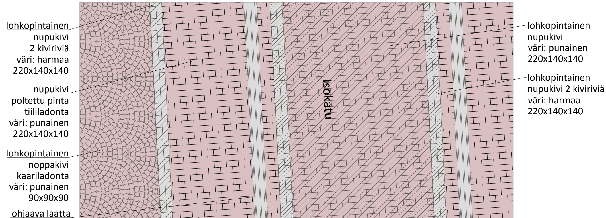
DETALJI 5: Isokadun ajoradan ja jalkakäytävien erottelu toriosuudella
